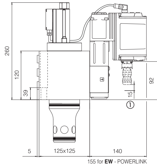
LIQZO-LEB-402 LIQZO-LES-402
