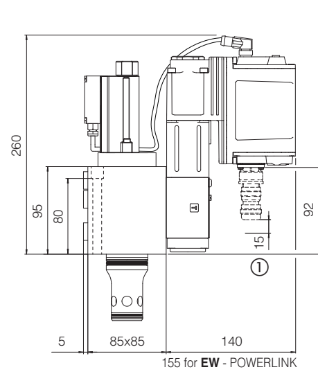
LIQZO-LEB-252 LIQZO-LES-252
