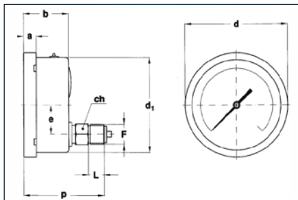
D-EX Manometry tylne ekscentryczne / Back connection excentric
